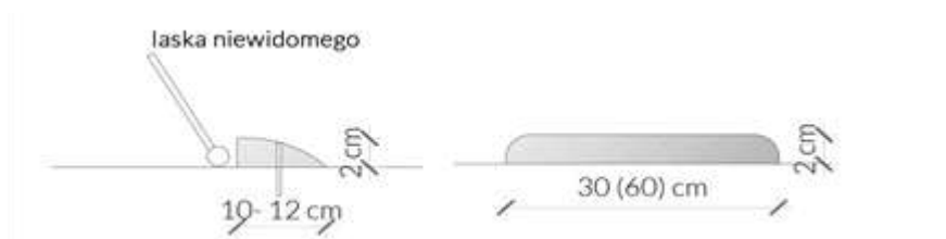
Rys. D3 – Profil rozdzielający ruch rowerowy od pieszego. Sygnalizujący koniec ciągu pieszego
